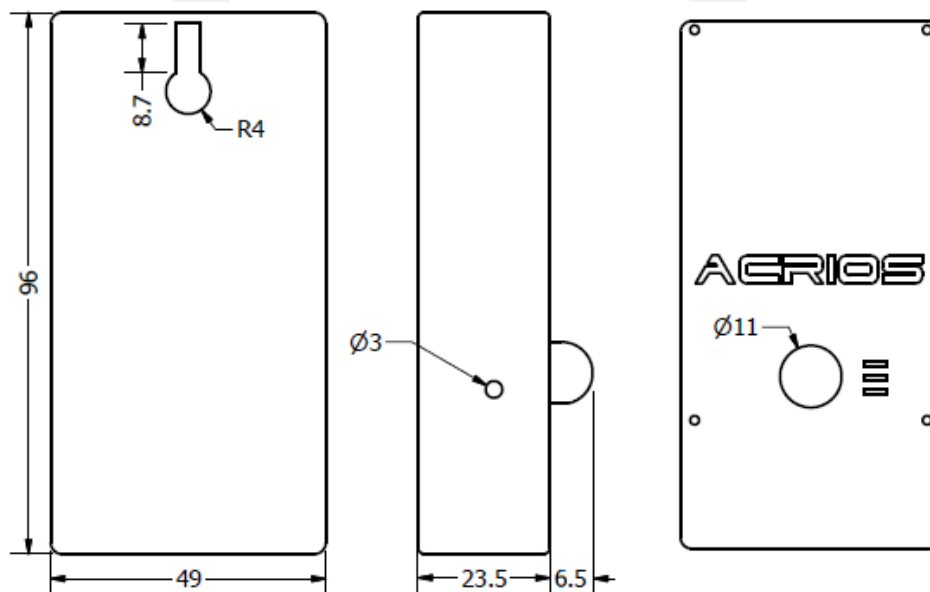
Obr. 1: Rozměry senzoru ACR-M-L-002
