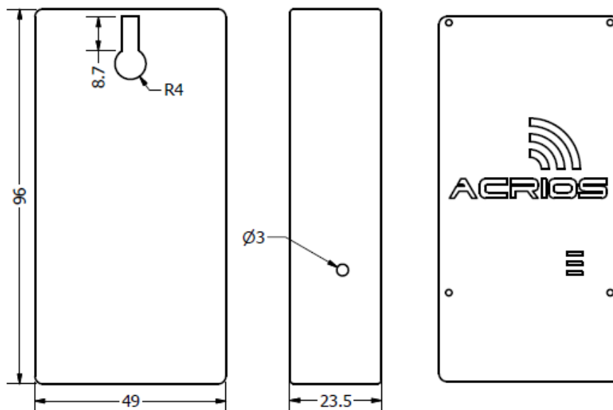
Obr. 1: Rozměry senzoru ACR-TH-L-001
