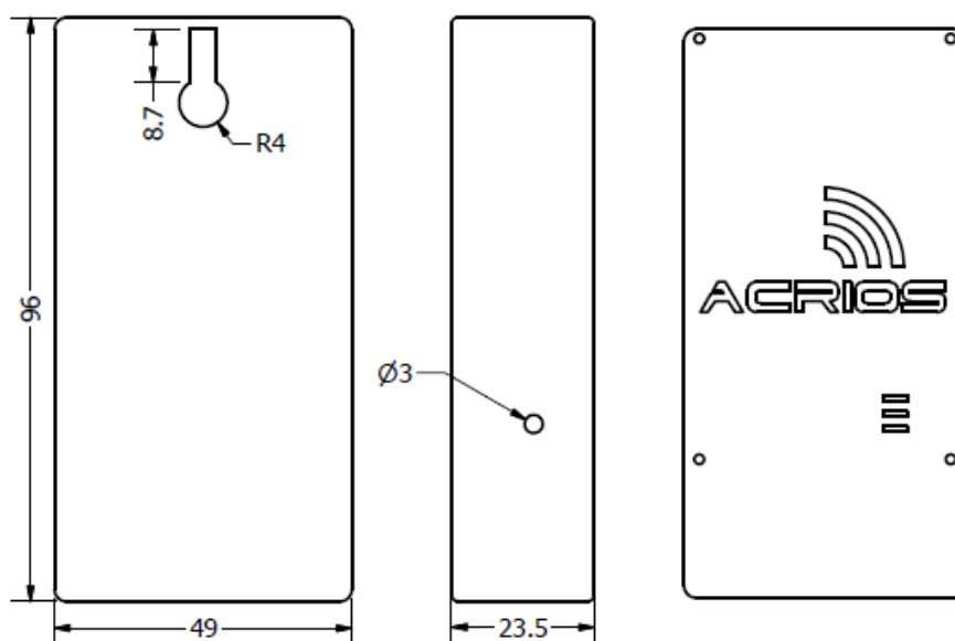
Obr. 1: Rozměry senzoru ACR-TH-L-002
